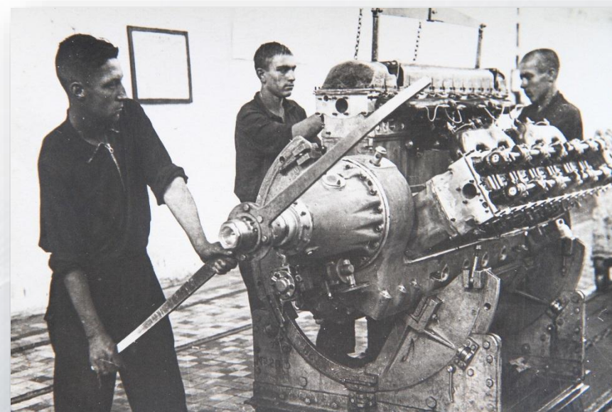
Сборка двигателя на заводе №24 им. Фрунзе
